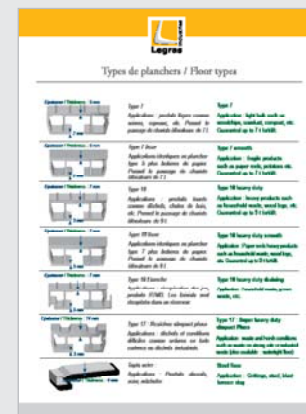
Bodenprofil Typen FMA®
